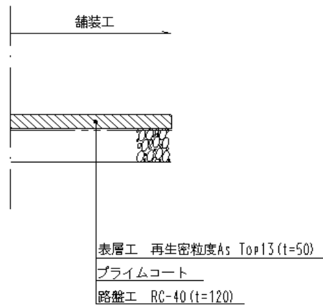
計画標準断面図
