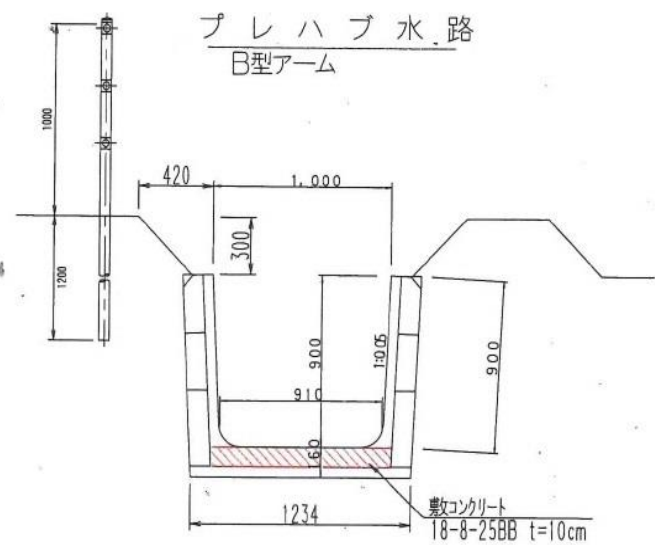
計画標準断面図
