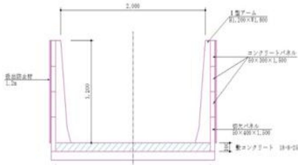
計画断面図
