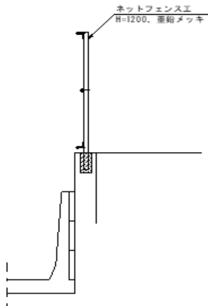
計画断面図
