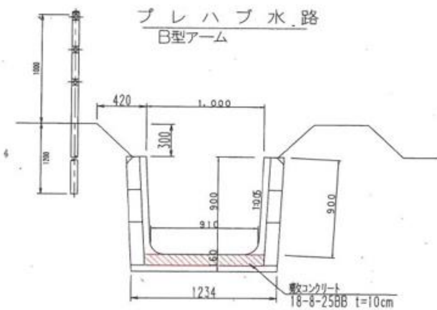
計画断面図
